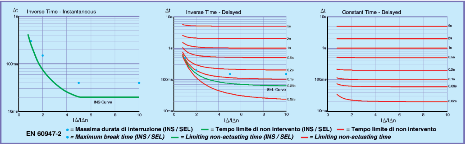
Figura 3 - Curve di intervento a tempo inverso e a tempo costante / Figure 3 - Inverse and constant time trip curves
