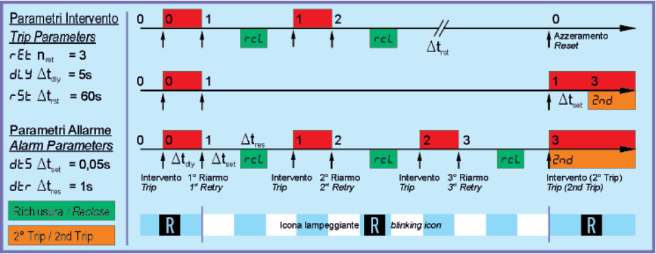
Figura 5 - Logica e temporizzazione riarmo automatico - funzioni Richiusura e 2° Trip Figure 5 - Automatic retry logic and timing - Reclose and 2nd Trip functions
