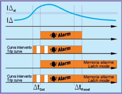
Figura 4 - Logica e temporizzazione allarme Figure 4 - Alarm logic and timing
