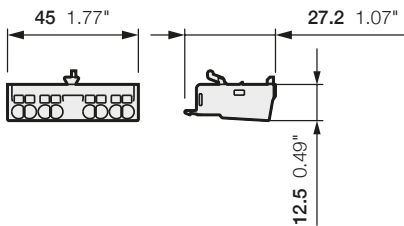
MAHN..FB
