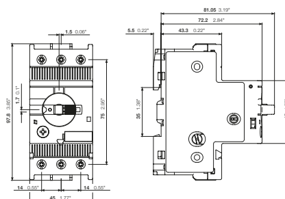
MBS32NH ≥ 12 A
