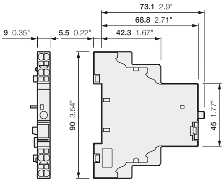
MAHN..LL
